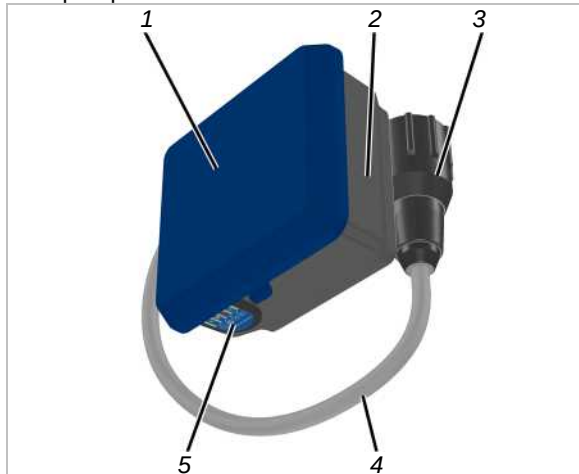
Receptor para ABURemote AC:
